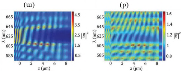
Նկ. 2. Լույսի տեղայնացման սպեկտրերը ԽՀԲ -ի ուղղորդի z առանցքի երկայնքով ուժեղ ( u ) և թույլ ( p ) դիֆրակտվող սեփական բևեռացումների համար: Մյուս պարամետրերը նույնն են, ինչ նկ. 1-ում են
