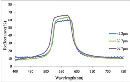
Նկ. 5. ԽՀԲ-ՆՀՊԹ-ԽՀԲ սեպան համակարգից փորձնականորեն գրանցված անդրադարձման սպեկտրերը բջջի երեք տարբեր հաստություններին համապատասխանող դիրքերում (47.3մկմ, 39.7մկմ, 32.7մկմ)
