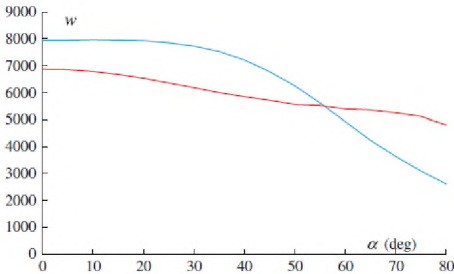
Նկ. 3. ԽՀԲ շերտում միջինացված լուսային էներգիայի խտության կախվածությունը անկման անկյունից կարճալիքային ( m = +1 կապույտ կոր) և երկարալիքային ( m = -1 կարմիր կոր) եզրերի մոդաների համար
