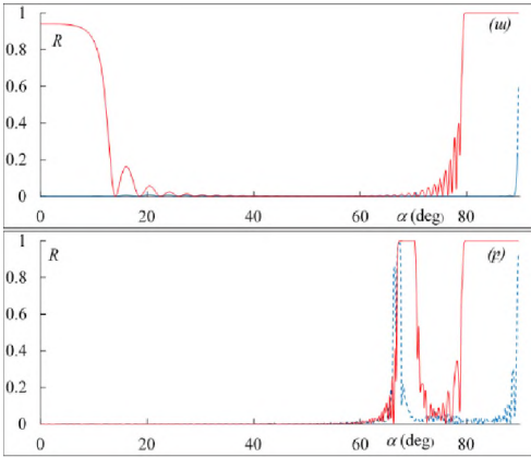
Նկ. 1. Անդրադարձման R գործակցի կախվածությունը անկման անկյունից ( u ) \lambda = \rho\sqrt{\epsilon_m} = 625 նմ և ( p ) \lambda = 225 նմ ալիքի երկարությունների համար: ԽՀԲ շերտի վրա ընկնող լույսի բևեռացումը համընկնում է առաջին (կարմիր կոր) և երկրորդ (կապույտ կոր) սեփական բևեռացումներին: ԽՀԲ շերտը ունի հետևյալ պարամետրերը՝ p=420 նմ, \epsilon_1=2.29 , \epsilon_2=2.143 , իսկ հաստությունը՝ d=20p
