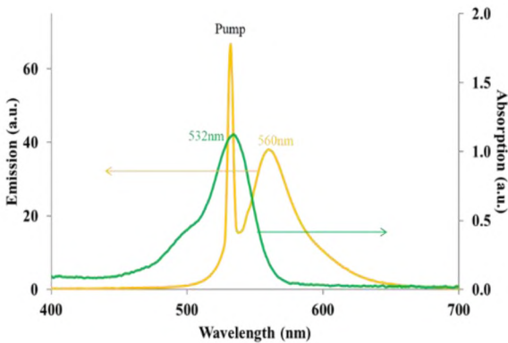
Նկ. 8. ՆՀՊԹ-ի կլանման և ճառագայթման սպեկտրը
